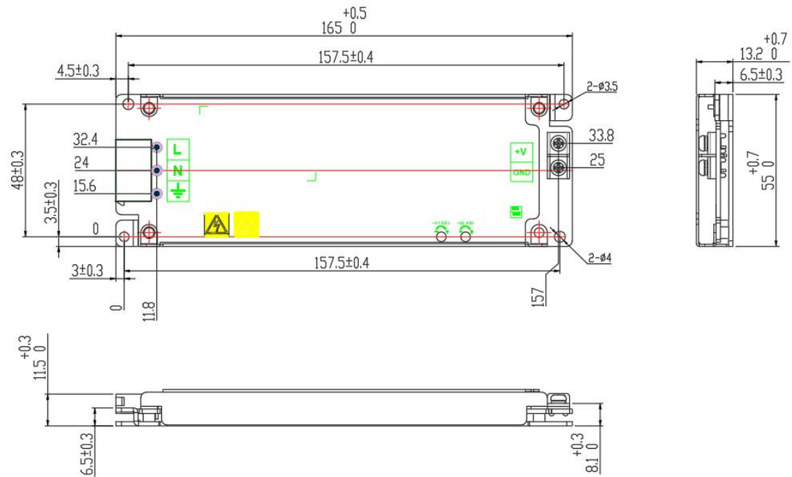
输入、输出端子定义及安装注意事项
